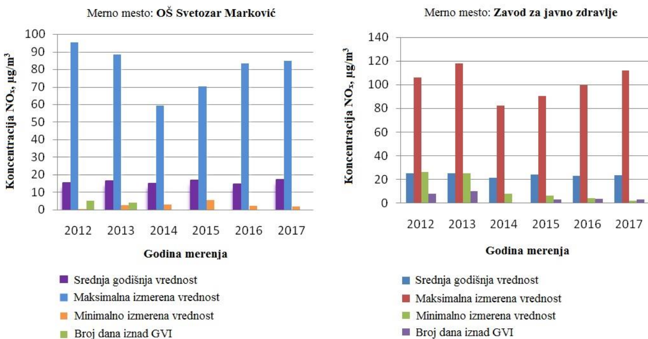
Slika 4. Grafički prikaz koncentracija azotnih oksida izmerenih na teritoriji grada Leskovca.
