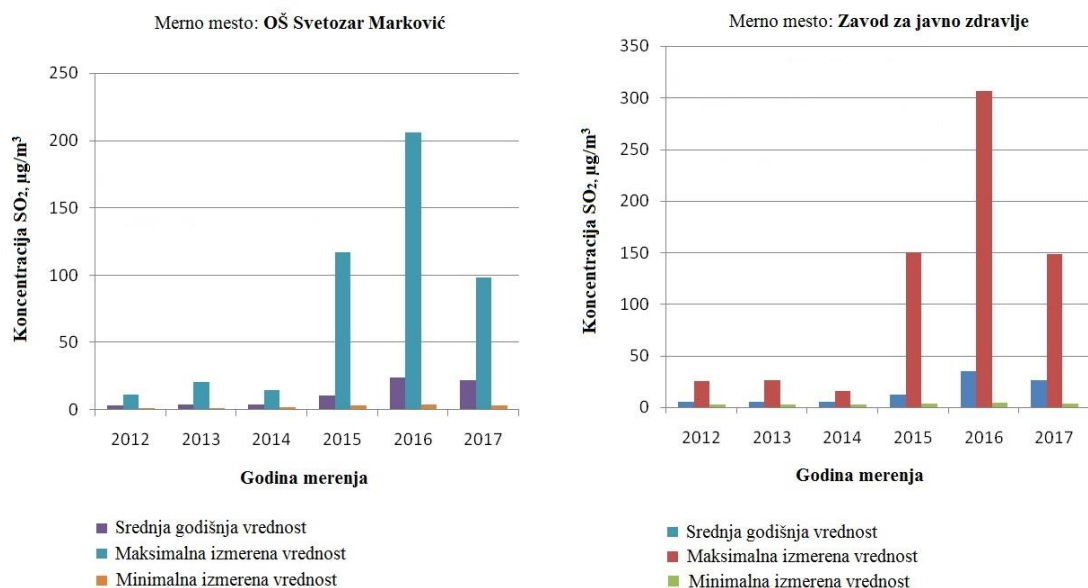
Slika 3. Grafički prikaz koncentracija \text{SO}_2 izmerenih u periodu od 2012. do 2017. godine na teritoriji grada Vranja.
