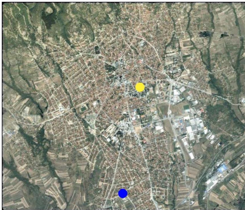
Slika 1. Merna mesta na teritoriji grada Leskovca: Zavod za javno zdravlje (●) i OŠ "Svetozar Marković" (●) [6]
