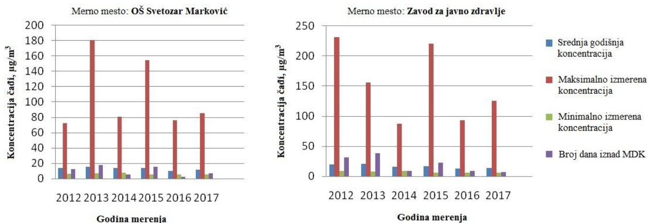
Slika 2. Trend kretanja koncentracija čadi na teritoriji grada Vranja u periodu od 2012. do 2017. godine.
